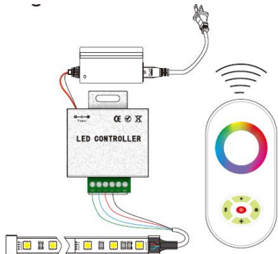
Схема підключення
